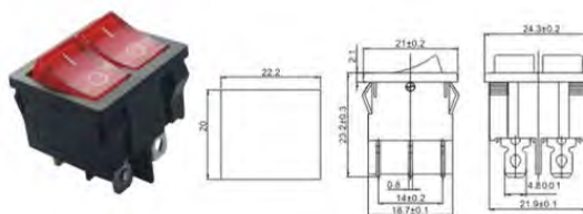
A-TOP1-6-2101 ON-OFF A-TOP1-6-2101N ON-OFF A-TOP1-6-2102 ON-ON
