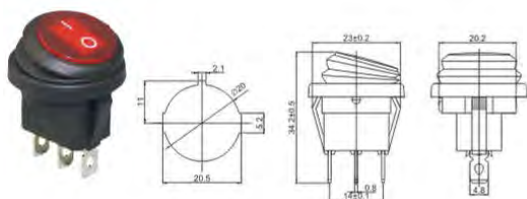
A-TOP1-8-102W ON-ON A-TOP1-8-103W ON-OFF-ON
